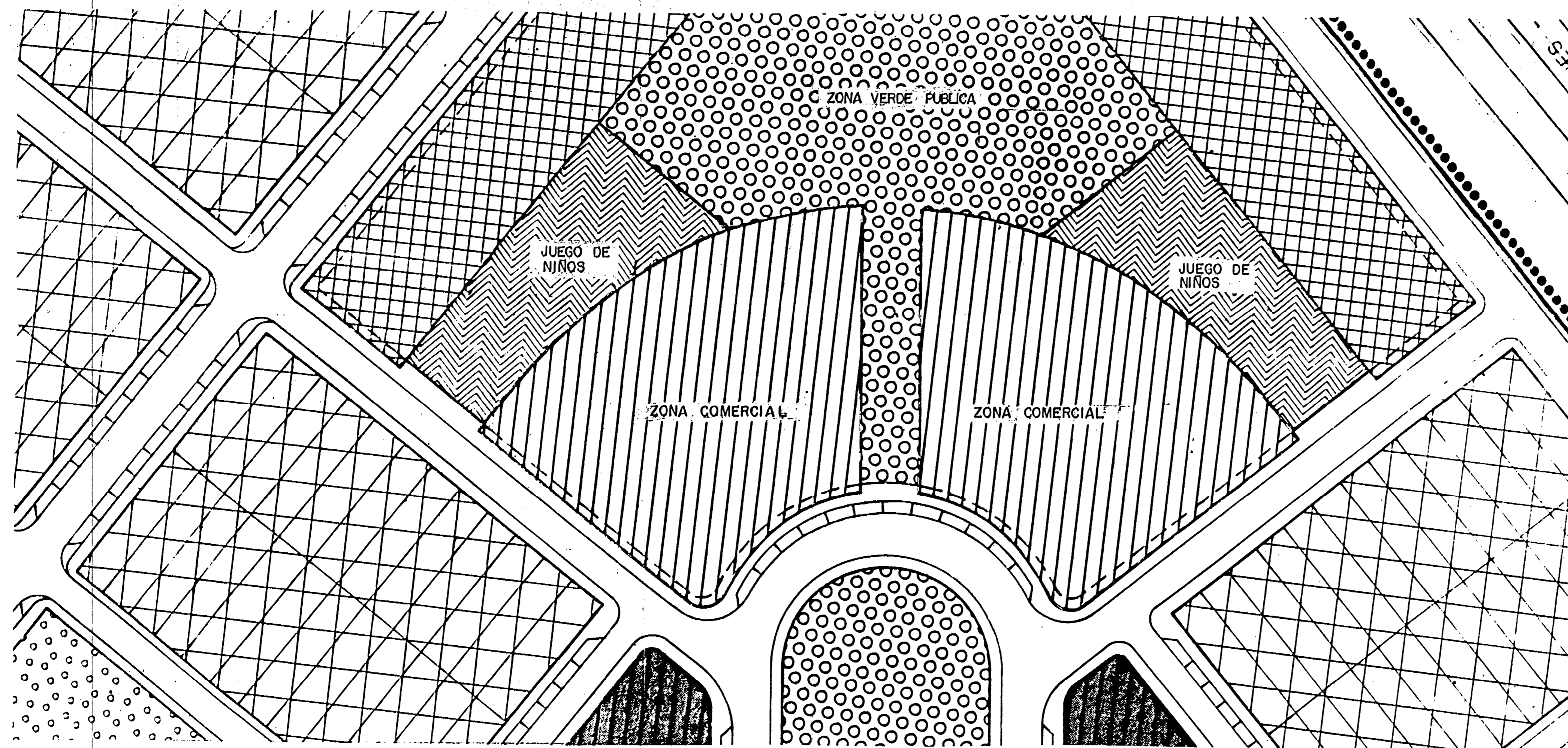
PLANO DE PLAN PARCIAL (DETALLE) 1/500
