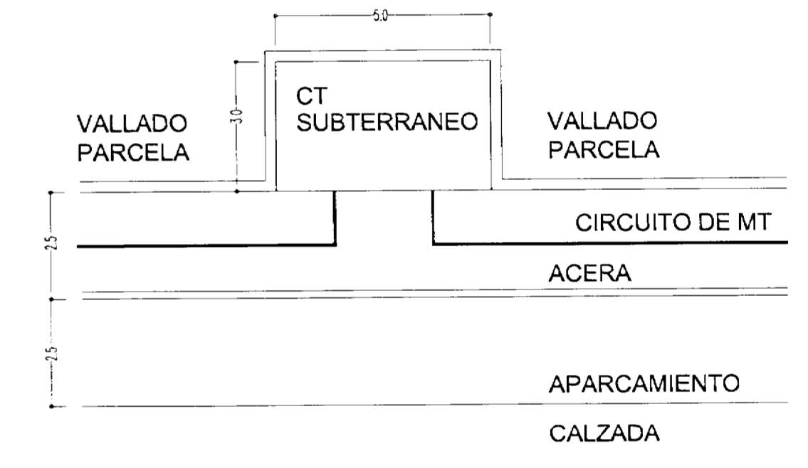
ESQUEMA DE POSICIÓN DE LOS CENTROS DE TRANSFORMACIÓN
