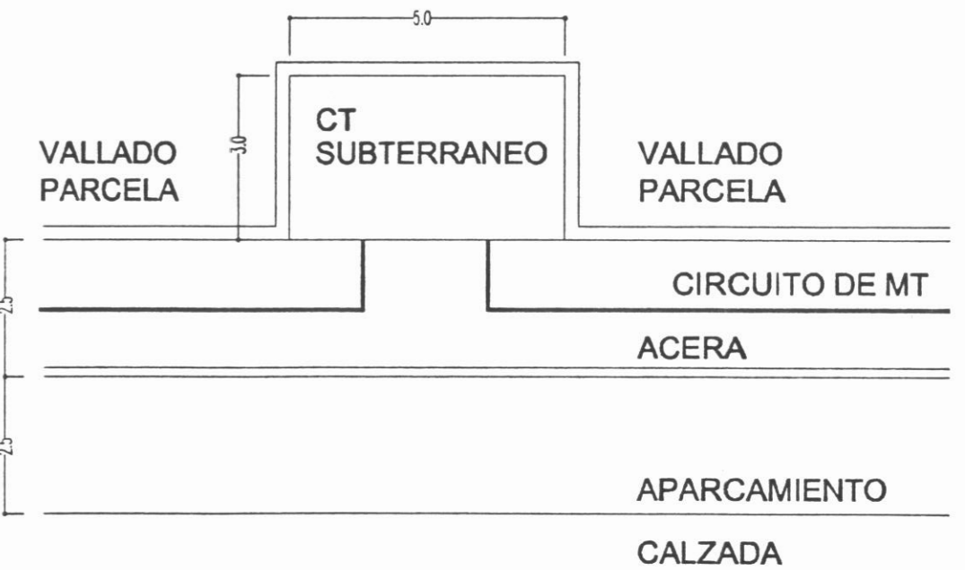
ESQUEMA DE POSICIÓN DE LOS CENTROS DE TRANSFORMACIÓN
